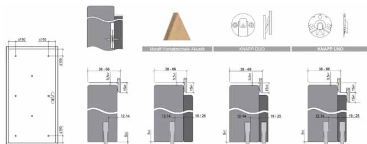
39 dB Rwp 40 dB Rwp 42 dB Rwp 43 dB Rwp
